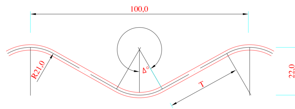
DETTAGLIO SEZIONE PIASTRA SCALA 1:1
