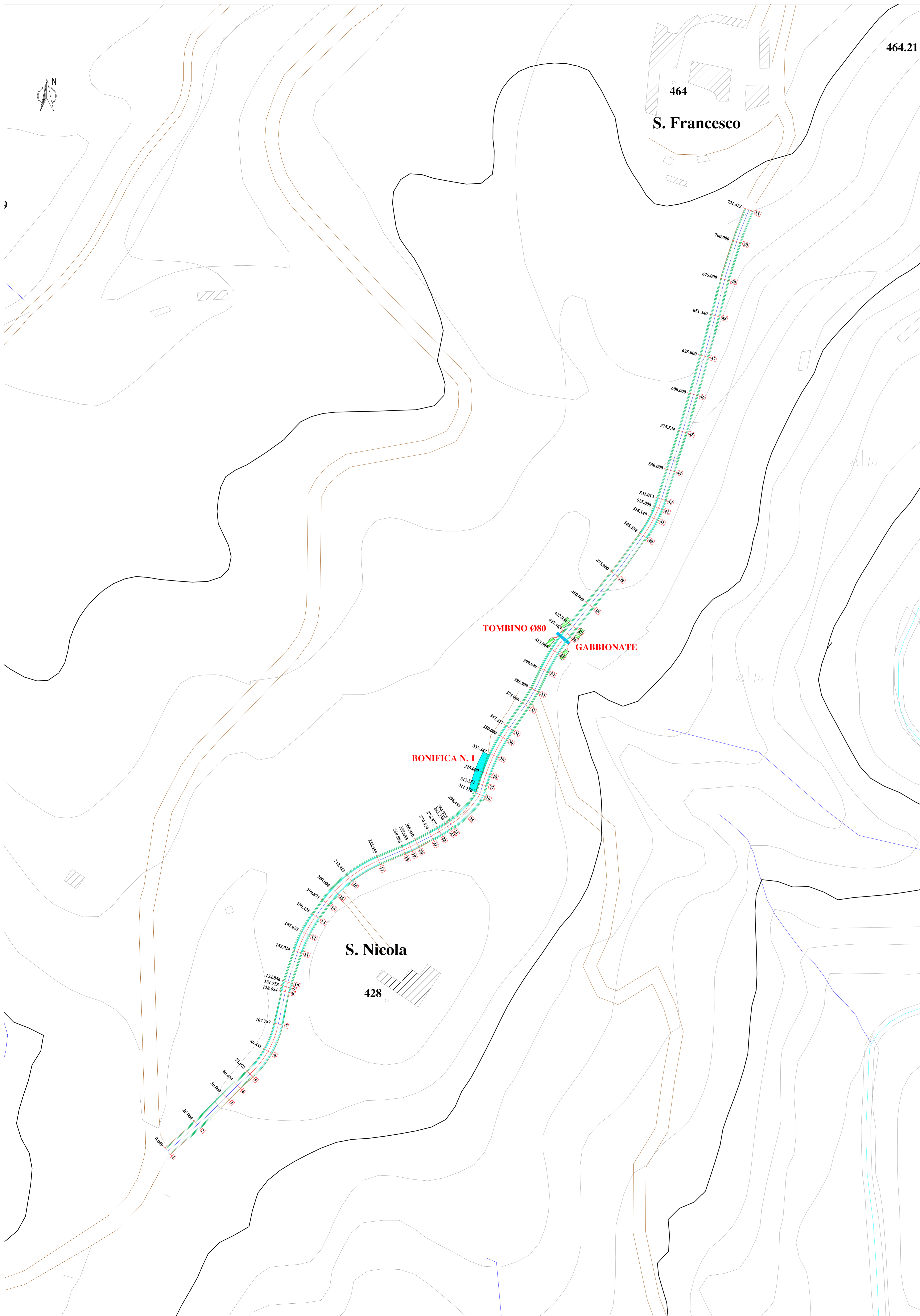
Strada Vicinale S.Nicola: Planimetria di Progetto scala 1:1000
