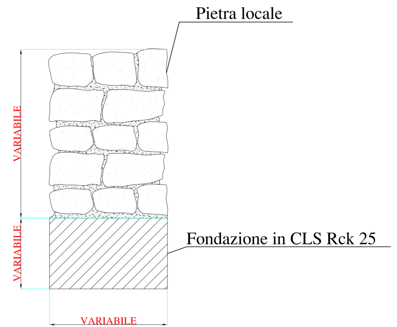
SEZIONE TIPO MURETTI IN PIETRA DA ESEGUIRE NEI LUOGHI E NELLE DIMENSIONI INDICATE DALLA D.L.
