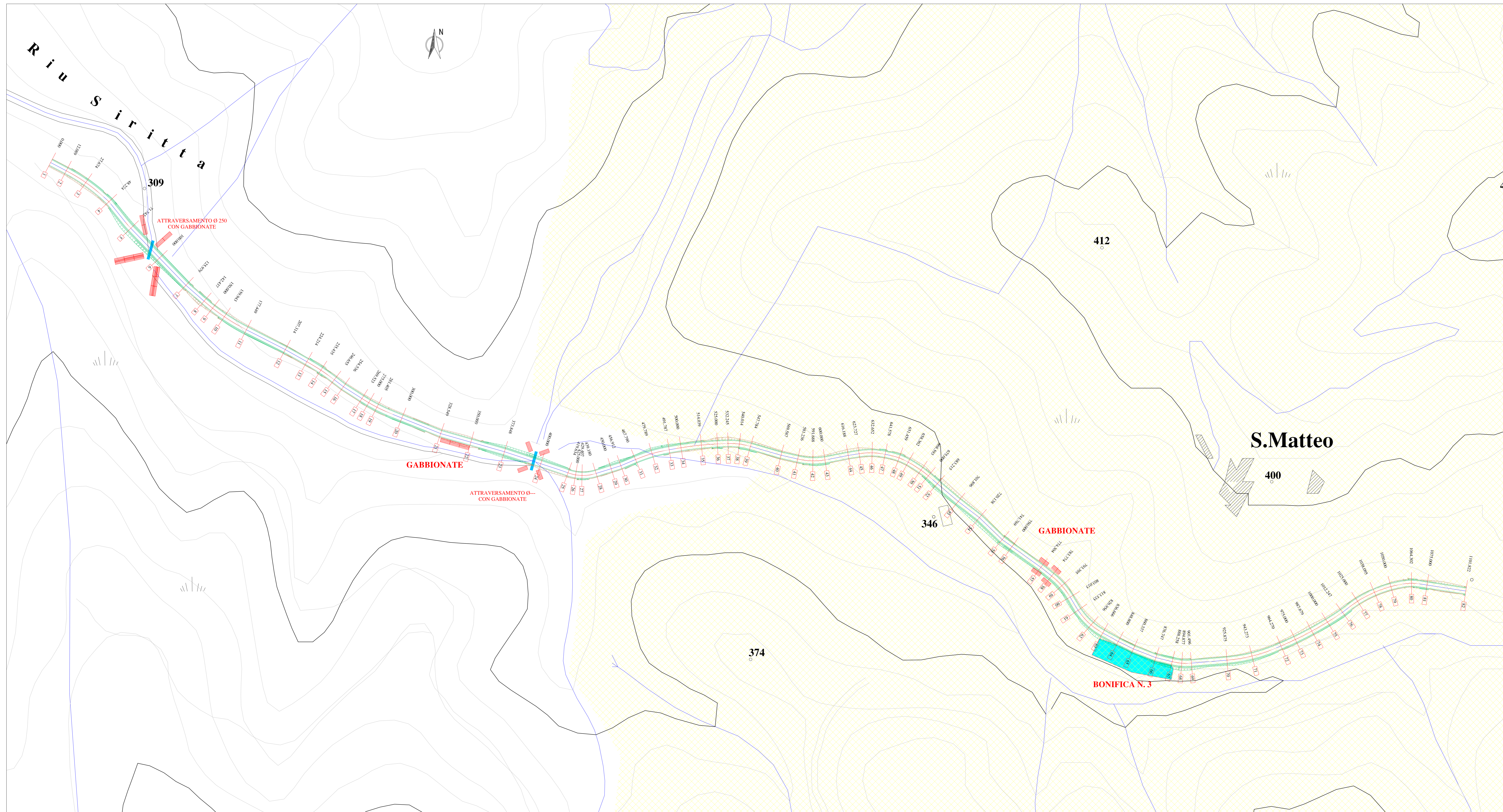
Strada Vicinale S.Matteo: Planimetria di Progetto scala 1:1000
