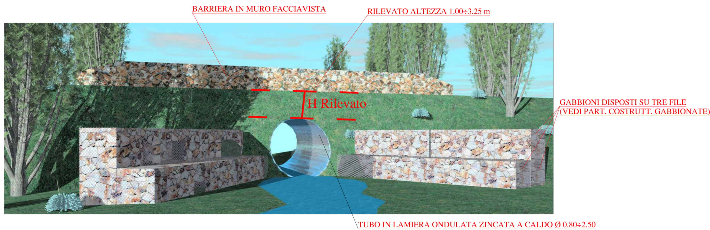
SCEMA TIPO DI ATTRAVERSAMENTO CON GABBIONI :VISTA MONTE
