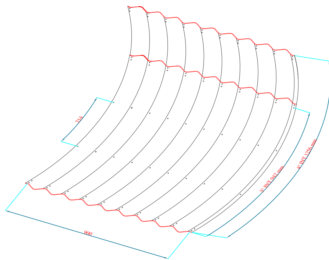
SOVRAPPOSIZIONE PIASTRE AD INTERASSE DI 314 mm
